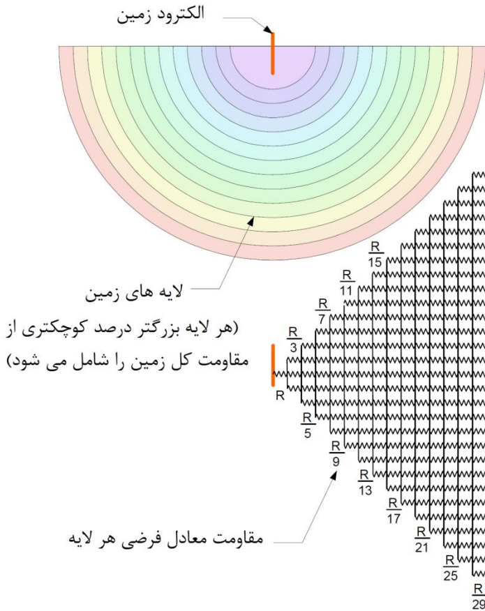
شکل (۱۷): مدار معادل پوسته‌های هم‌پتانسیل طرف یک الکتروود
